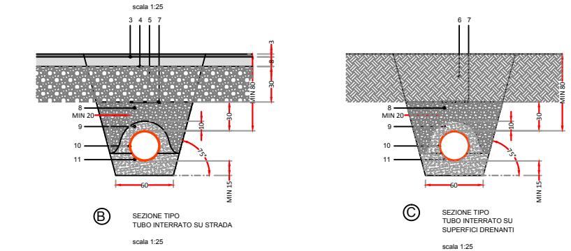
DETTAGLI ESECUTIVI
