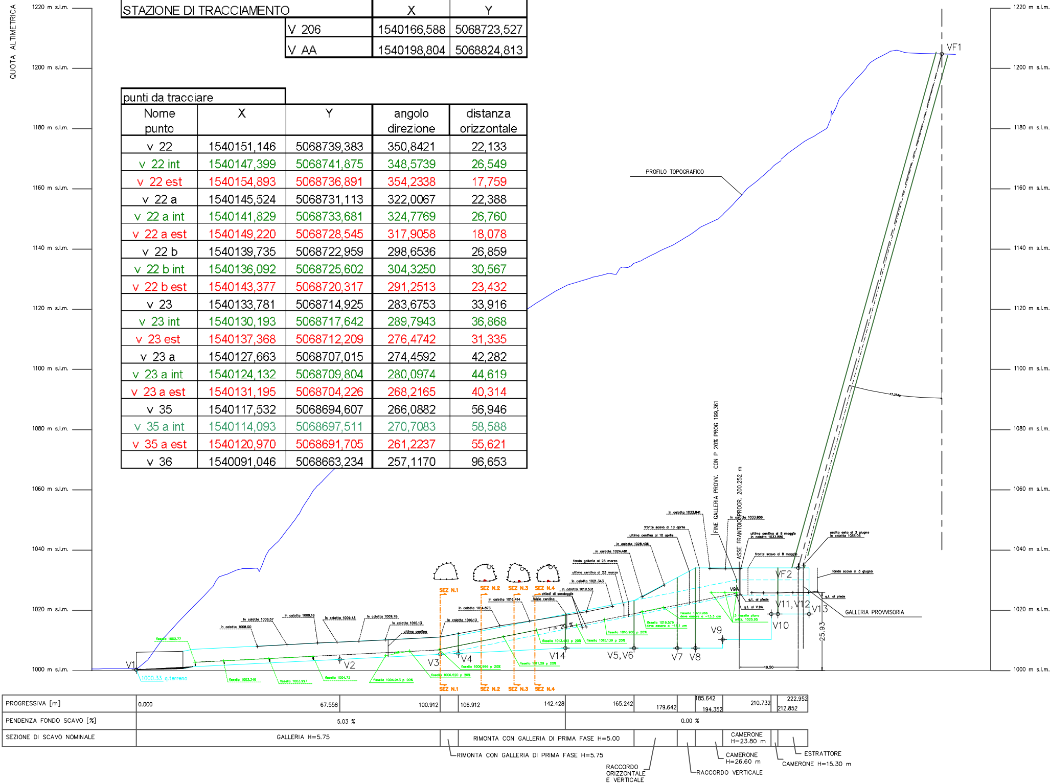
PROFILO ALTIMETRICO
